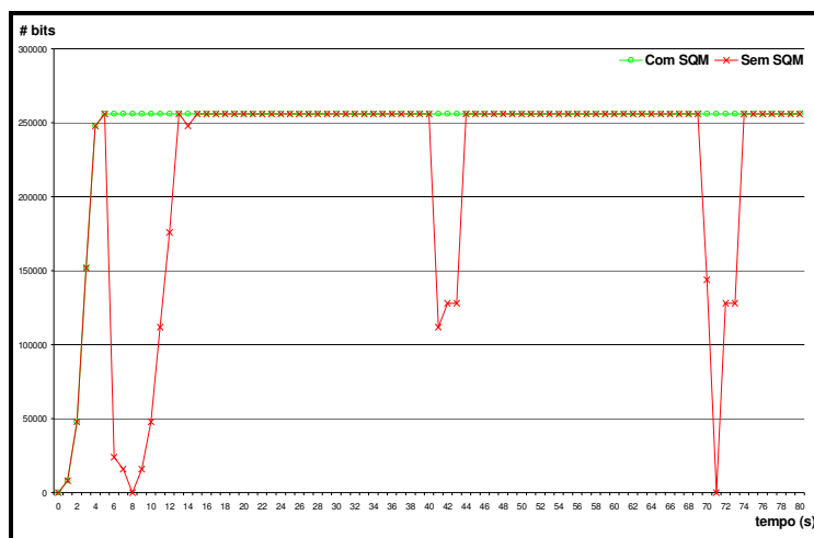
Figura 4 – Vazão do TCP Reno
